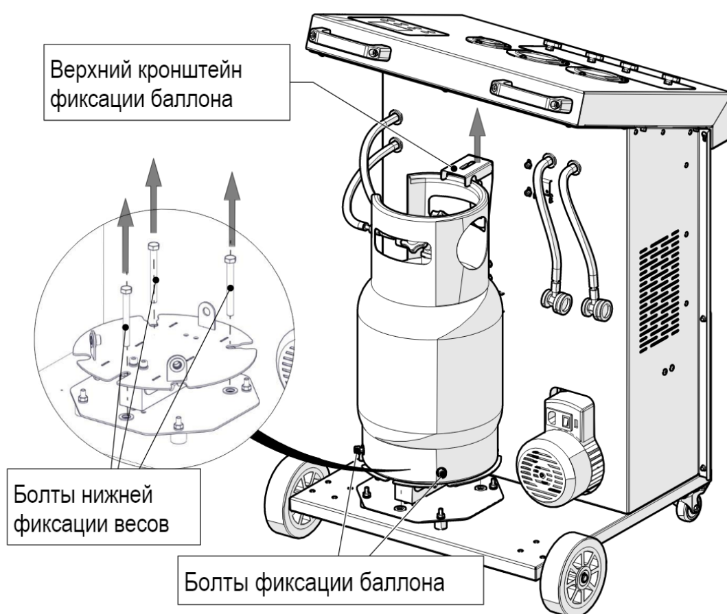
Рис. 5 Фиксация внутреннего бака
