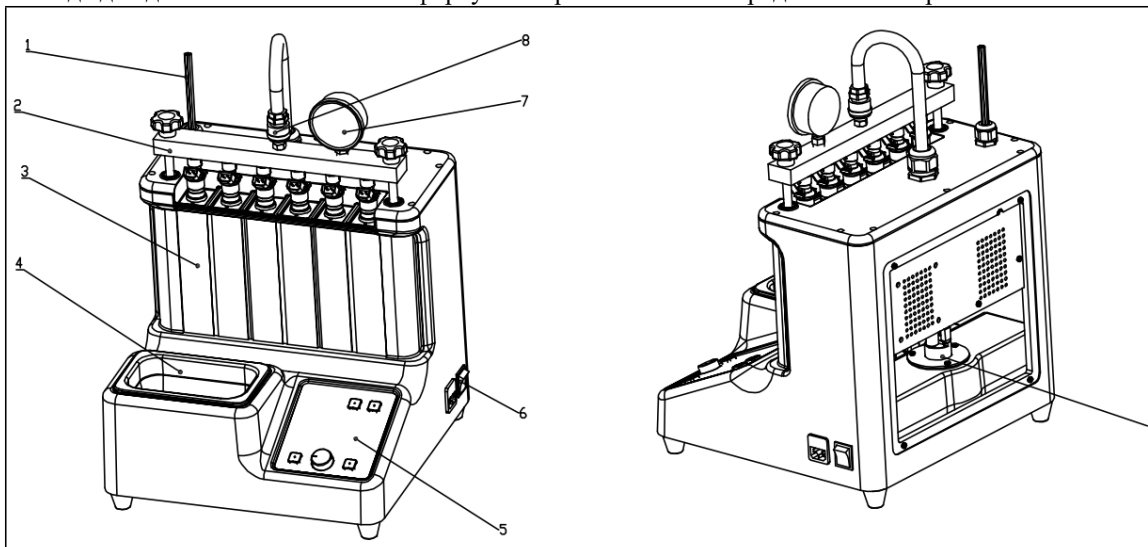
Рис. 2.1 Схема стенда модели CNC-603A
