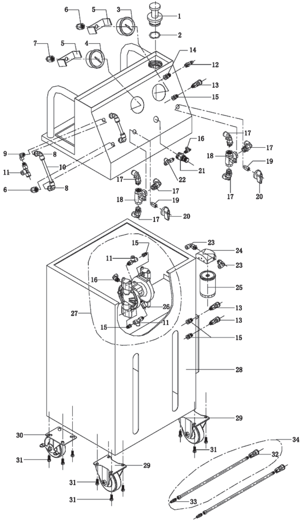
Рис.2 Устройство изделия
