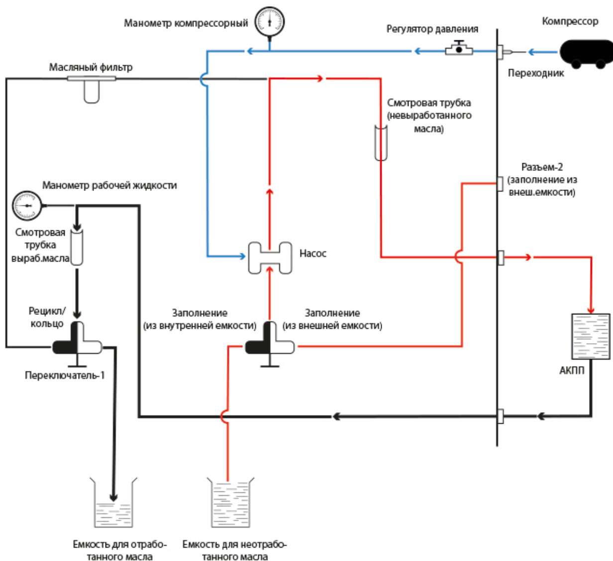
Рис.7 Общая схема цикла очистки
